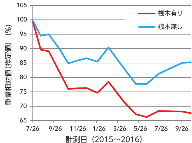
SPT計測で推定した丸太の重量の推移(70本の平均)
